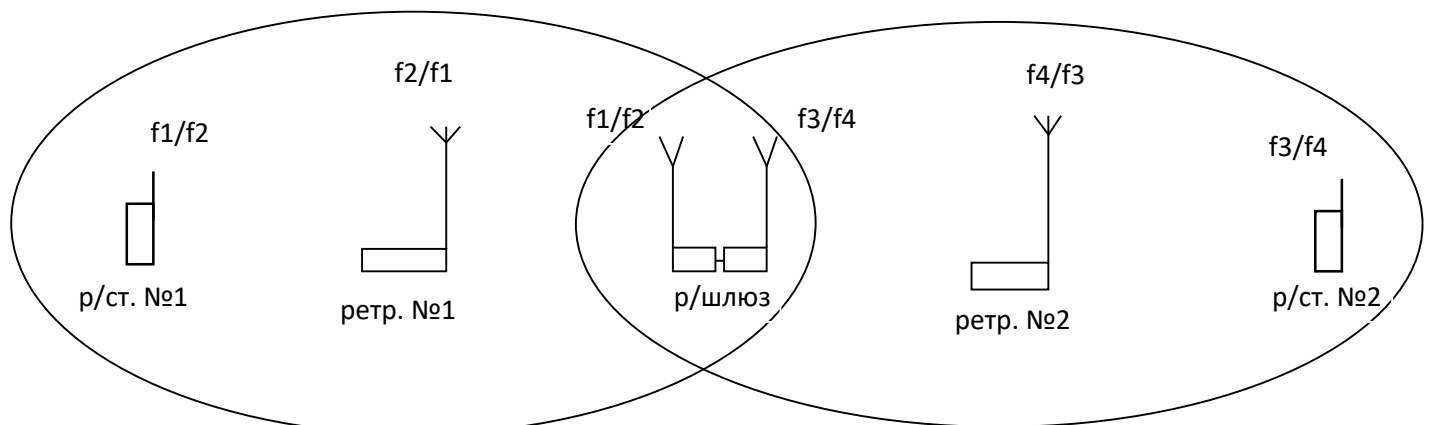
Малюнок 1. Схема організації зв'язку з використанням радіошлюза,
